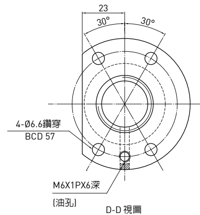
D-D視圖
