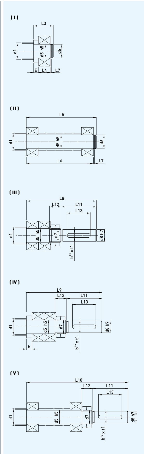
圖3.9 螺桿肩部型式
