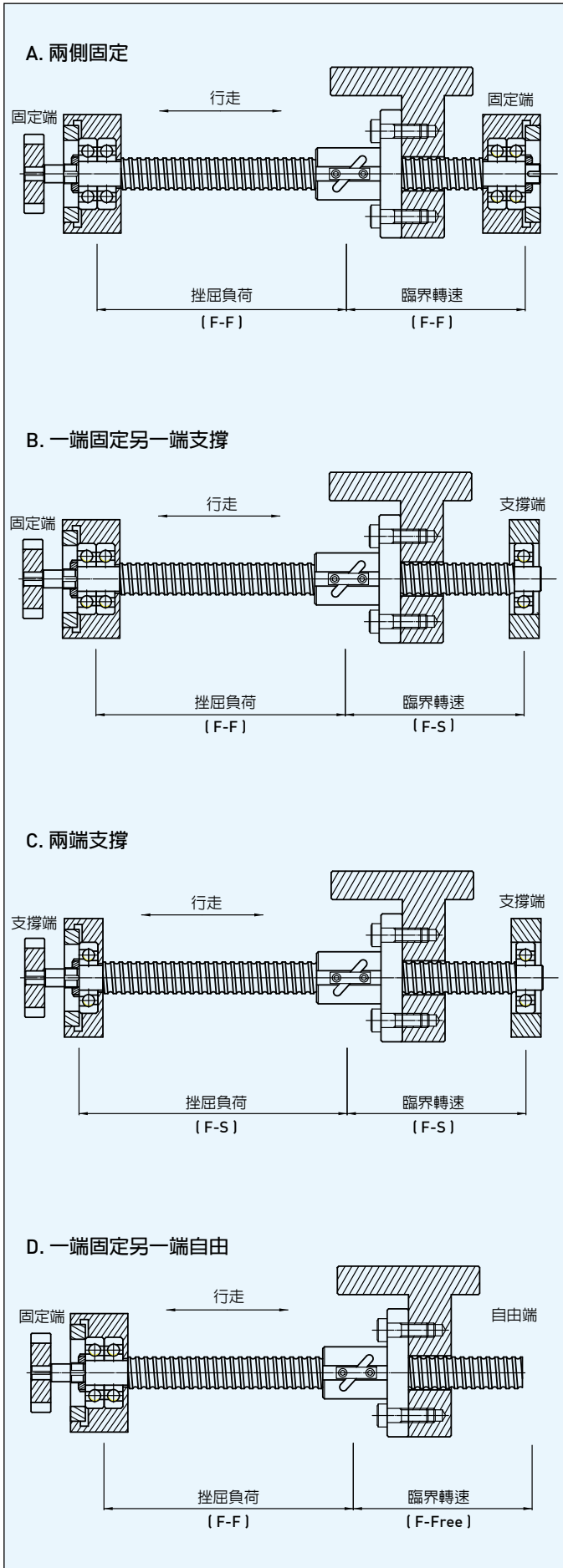
圖3.8 滾珠螺桿安裝實例
