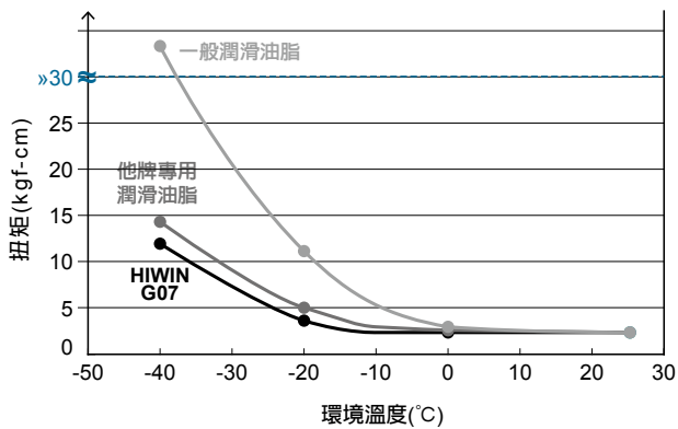
不同油脂啓動扭矩比較 @ -40 ^{\circ}\text{C}
