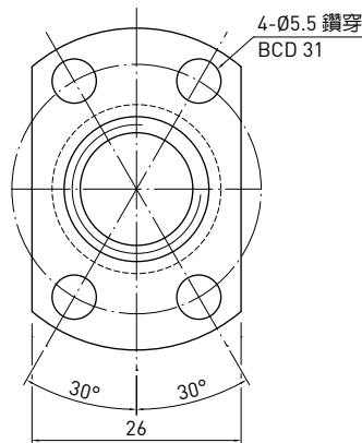
D-D 視圖
