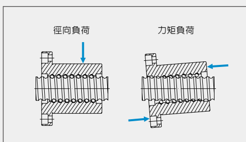
圖4.3(a) 引起非均衡負荷之原因：支撐軸承與螺帽法蘭組裝不同心，直角度不佳的引導面，螺帽安裝偏差或角度不準確。
