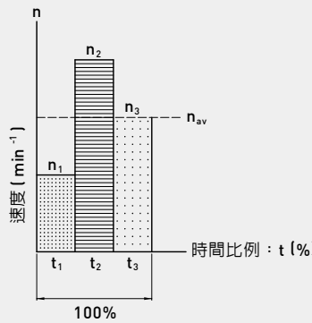
圖 4.22 等效速度
