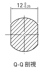
Q-Q 剖視
