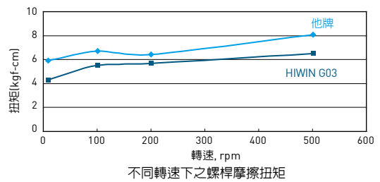
不同轉速下之螺桿摩擦扭矩
