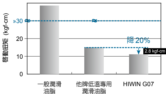
不同油脂啓動扭矩比較 @ -40 ^{\circ}\text{C}
